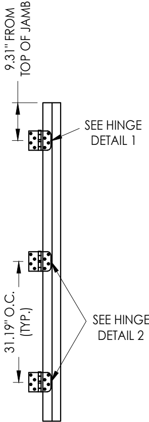
HINGE JAMB
